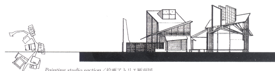
Painting studio section / 絵画アトリエ断面図
